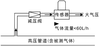
安装方式 1
