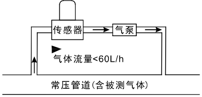
安装方式 2
