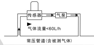
安装方式 2
